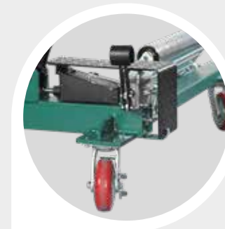
Fotmanövrerad växling mellan lyft- och sänkverkan.
